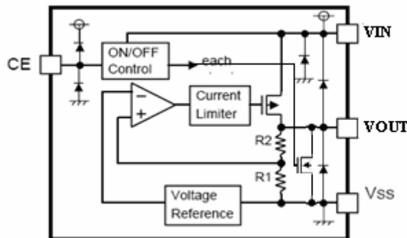
图 1 HM1134功能框图
