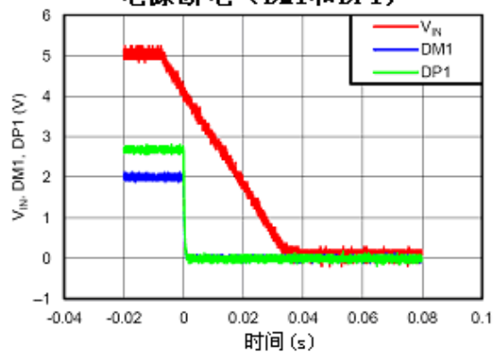
电源断电 (DM1和DP1)
