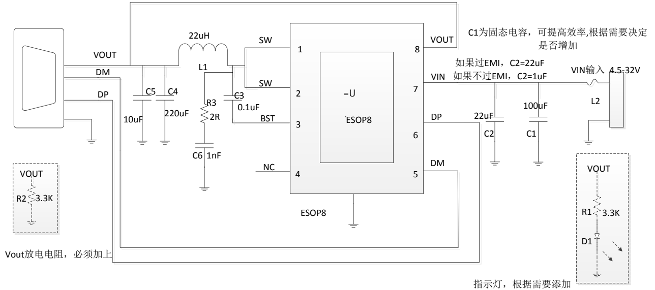
图5 =U 输出应用原理图
