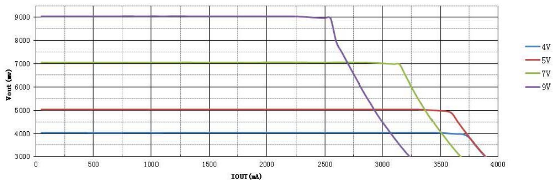
VIN=12V输出电压曲线
