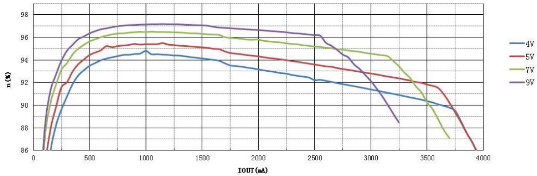
VIN=12V效率曲线
