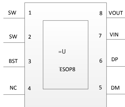
图 2 HM1597 引脚图
