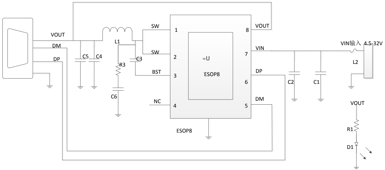
图 1 HM1597 简化应用原理图
