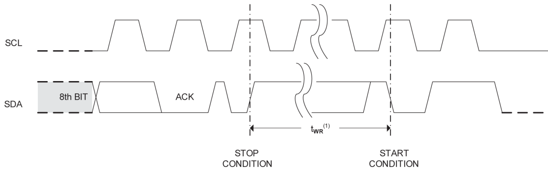
图 2. 总线时序
