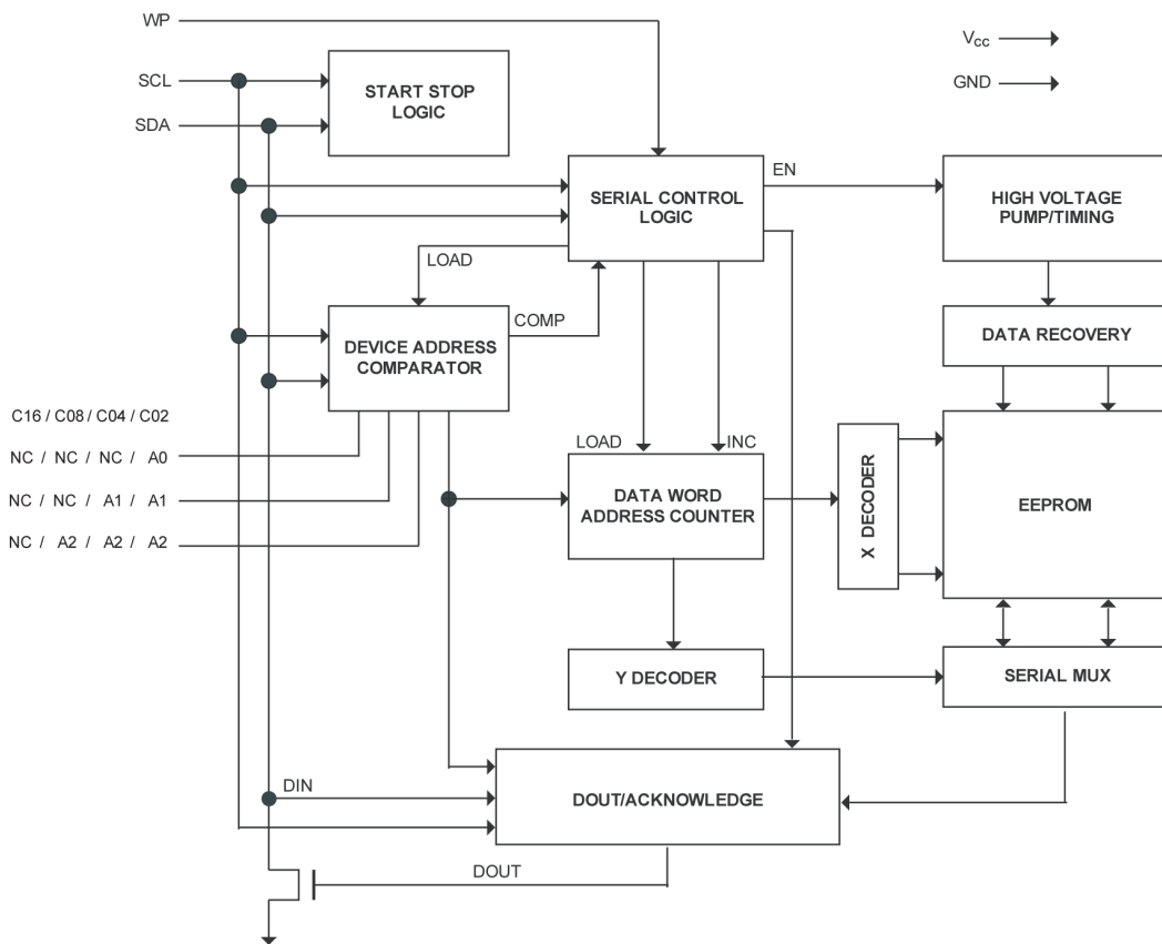
图 1. 框图
