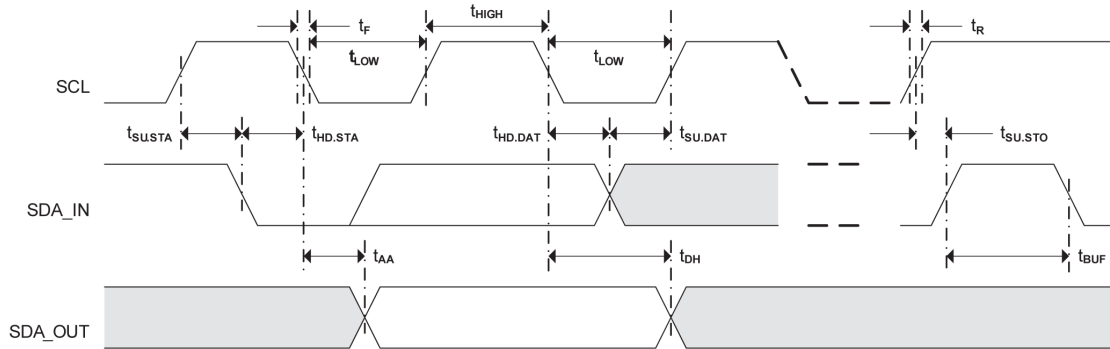
图 2. 总线时序
