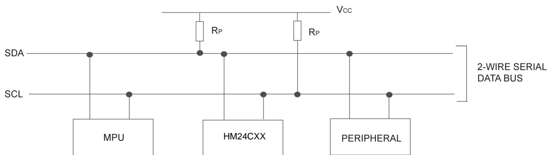
图 4. 典型两线总线配置
