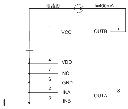
PMOS 体二极管导通电压测试原理图
