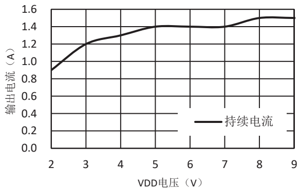
输出电流随VDD电压变化曲线
