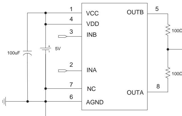
时间参数测试原理图
