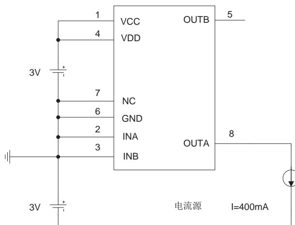
NMOS 体二极管导通电压测试原理图
