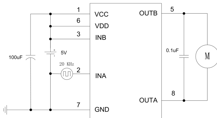
Time parameter test schematic
