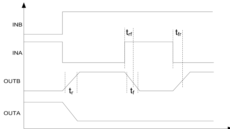
Time parameter definition
