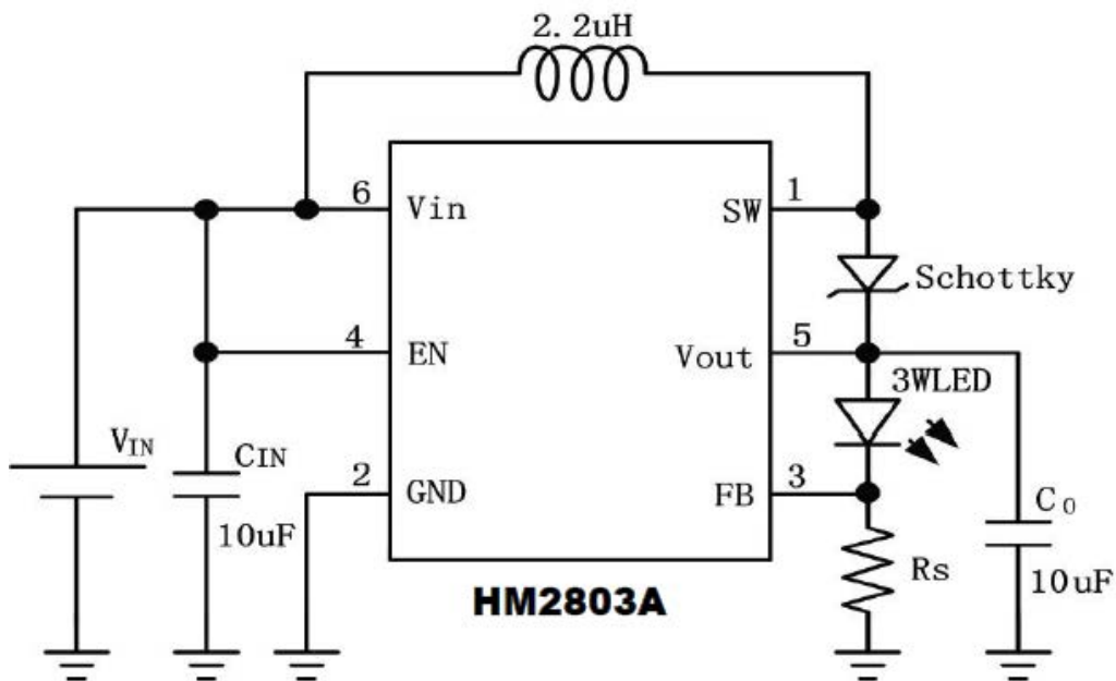
图 3. 典型应用电路
