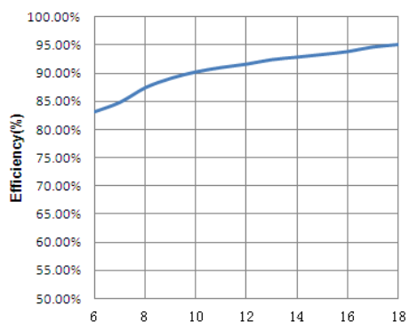
效率 VS. 输入电压(6 颗 LED)
