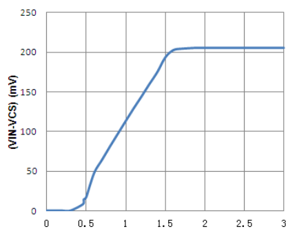
( V_{IN}-V_{CS} ) 电压 VS. ADJ 电压
