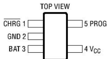
SOT23-5 封装
