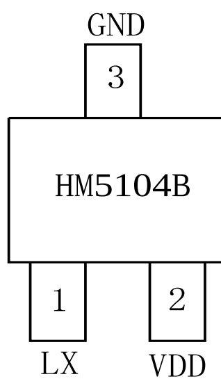
SOT23-3
