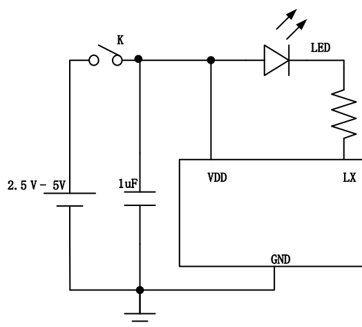
图 1. 典型应用电路
