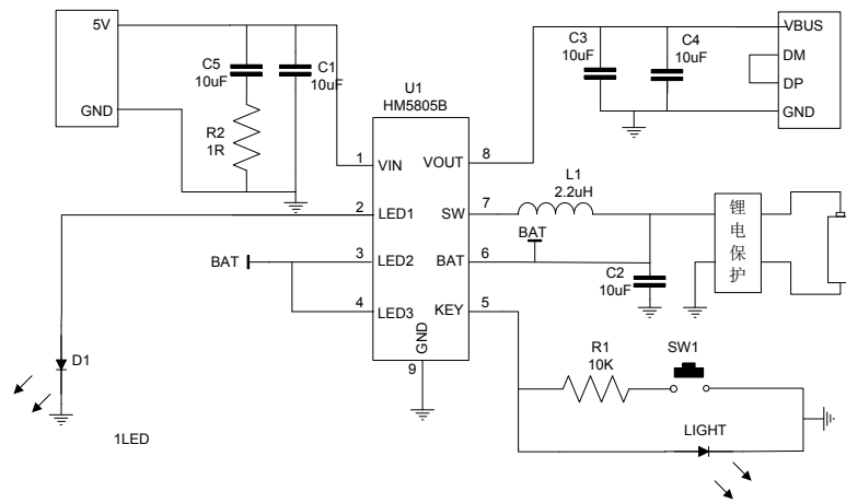
1LED 电量指示典型应用原理图
