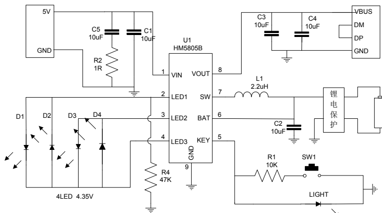
4.35V 电池供电典型应用原理图
