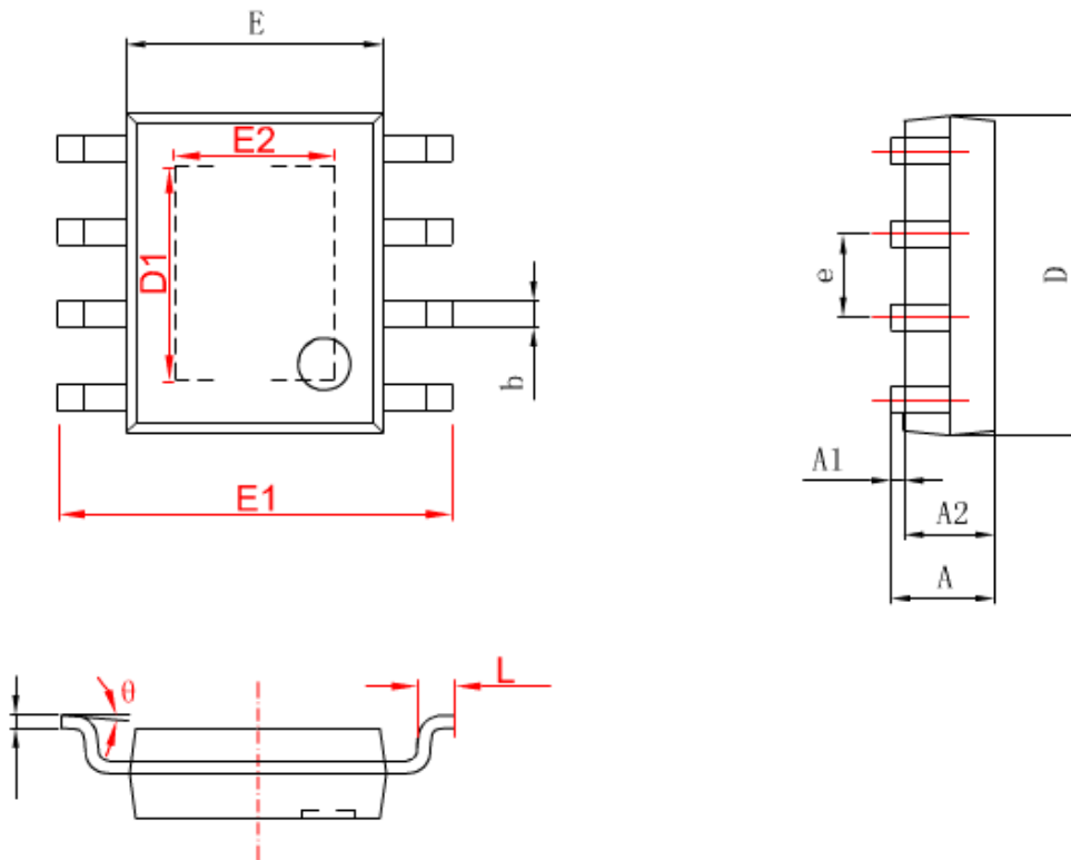
ESOP8 封装信息
