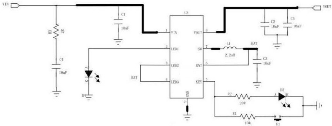
图 10 1LED 电量显示典型应用原理图
