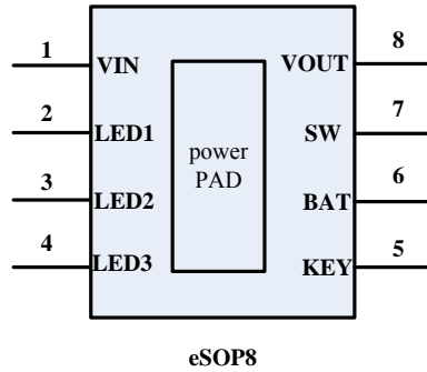
图 2 HM5905B-3 引脚图
