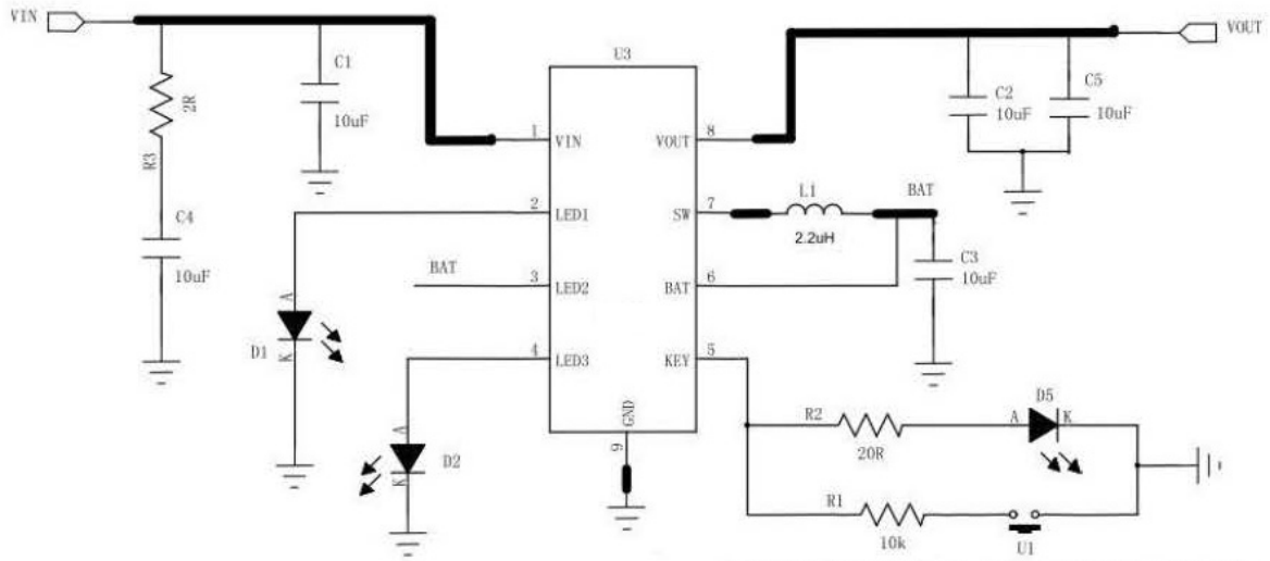
图 9 2LED 电量显示典型应用原理图
