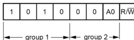
图10 HM8563 的器件地址字节的组成
