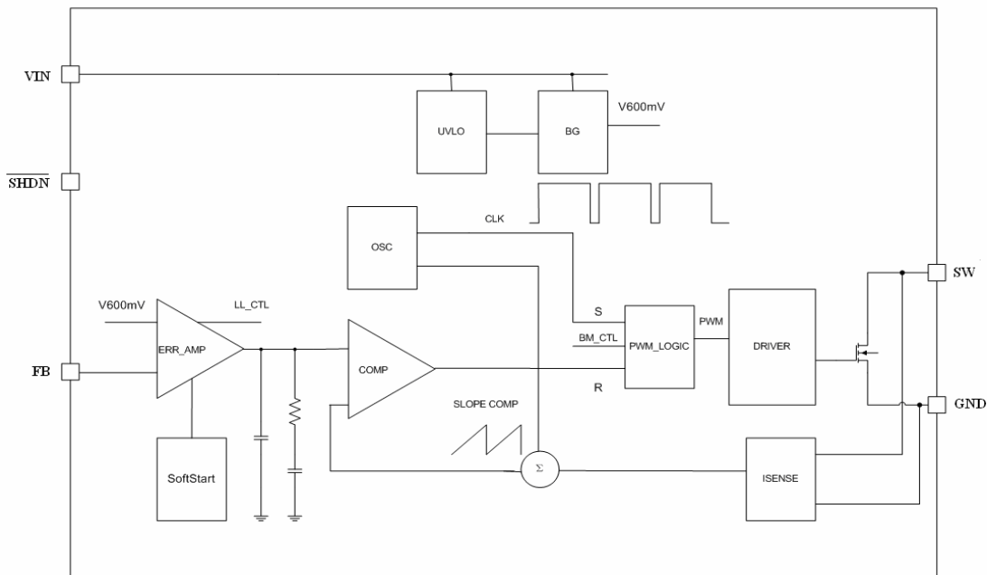
图 3 功能框图
